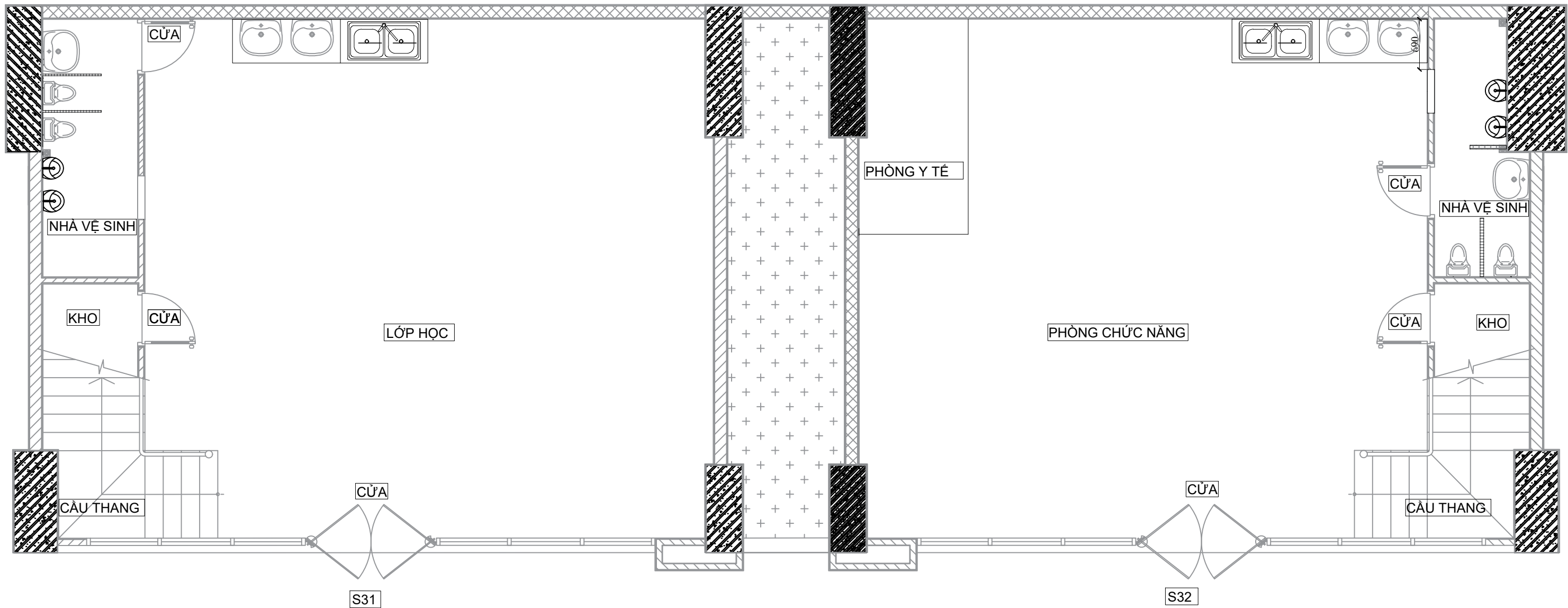
MẶT BẰNG TẦNG TRỆT
